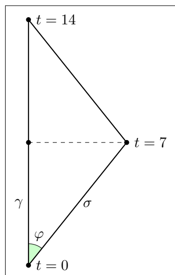
Abbildung 3.5: Das Zwillingsparadoxon
